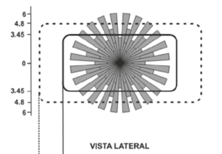
OSC20-MOW/ODC20-MOW Campo de visión en metros
