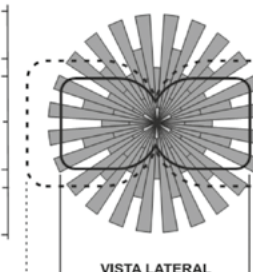
OSC10-MOW/ODC10-MOW Campo de visión en metros
