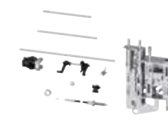
Enclavamiento mecánico
